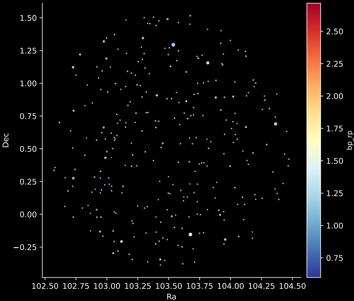
GALAH DR4 Field: [-4] Stars: 298
