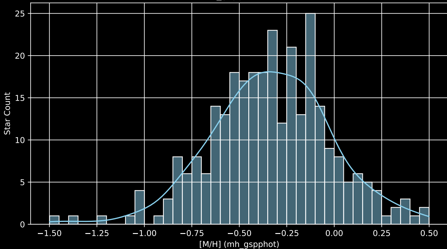
GALAH DR4 Field: [-4] [M/H] (mh_gspphot) (n= 292)
